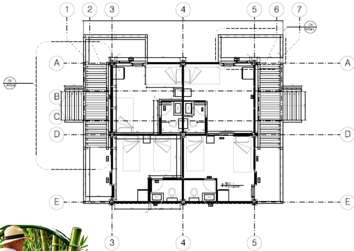
Planta Arquitectónica 1r Piso Escala 1:50
